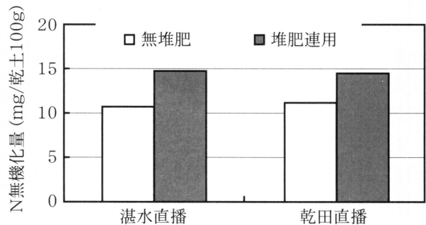
図3. 作付け後の作土の窒素無機化量（風乾土4週）
