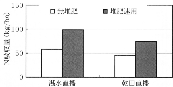
図2. 無窒素栽培区における黄熟期窒素吸収量
